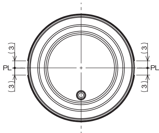
(印刷範囲) PLに対して前後3mmずつ開ける
